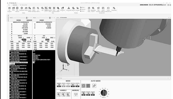
ゼロスダイナミックポストによるシミュレーション
